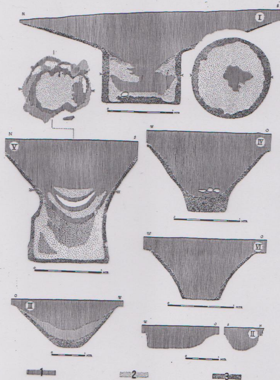
Abb. 7. Querschnitte der Opfergruben des Alkhūgels in Strazde (Legende: 1 — schwarze Füllerde, 2 — hellbraune Füllerde, 3 — dunkelbraune Kiesschicht).
