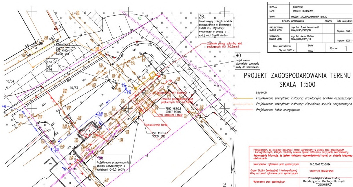
59. attēls. Projekta rasējums (avots: Gdańsk University of Technology).
