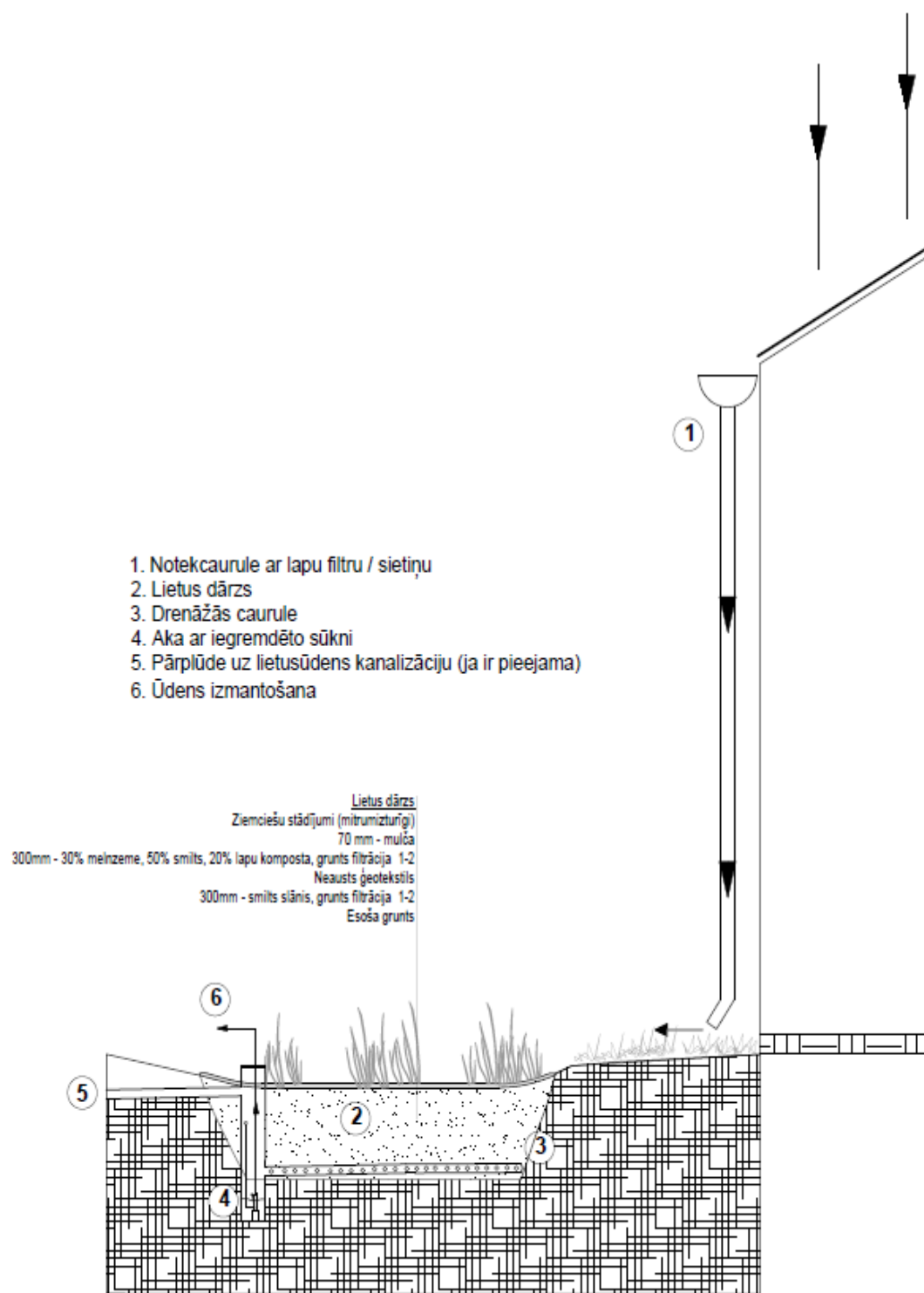
90. attēls. Shematisks piemērs risinājumam lietus ūdens izmantošanai laistīšanai ar uzkrāšanu lietus dārzā.
