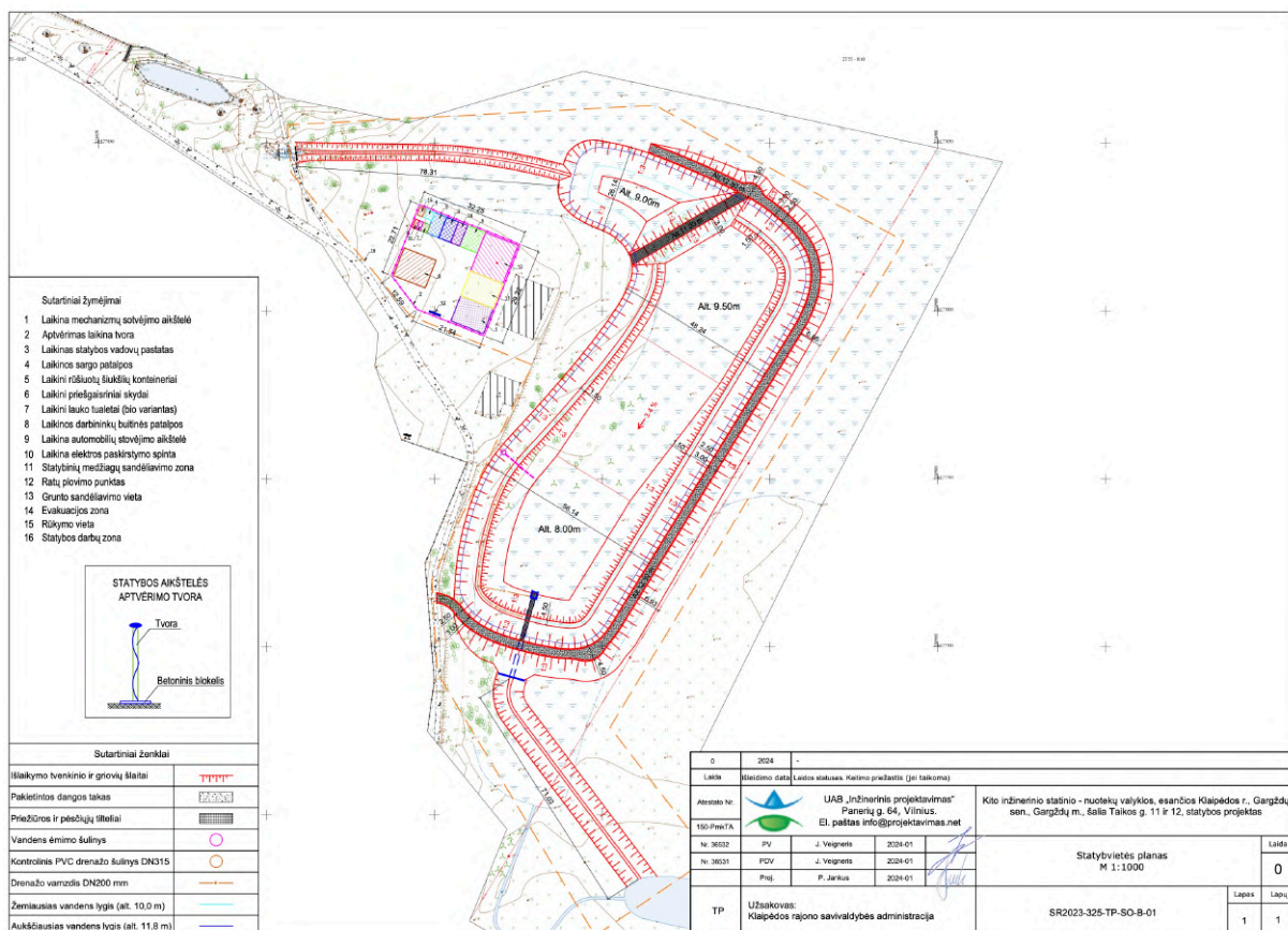
69. attēls. Dīķa rasējums.
