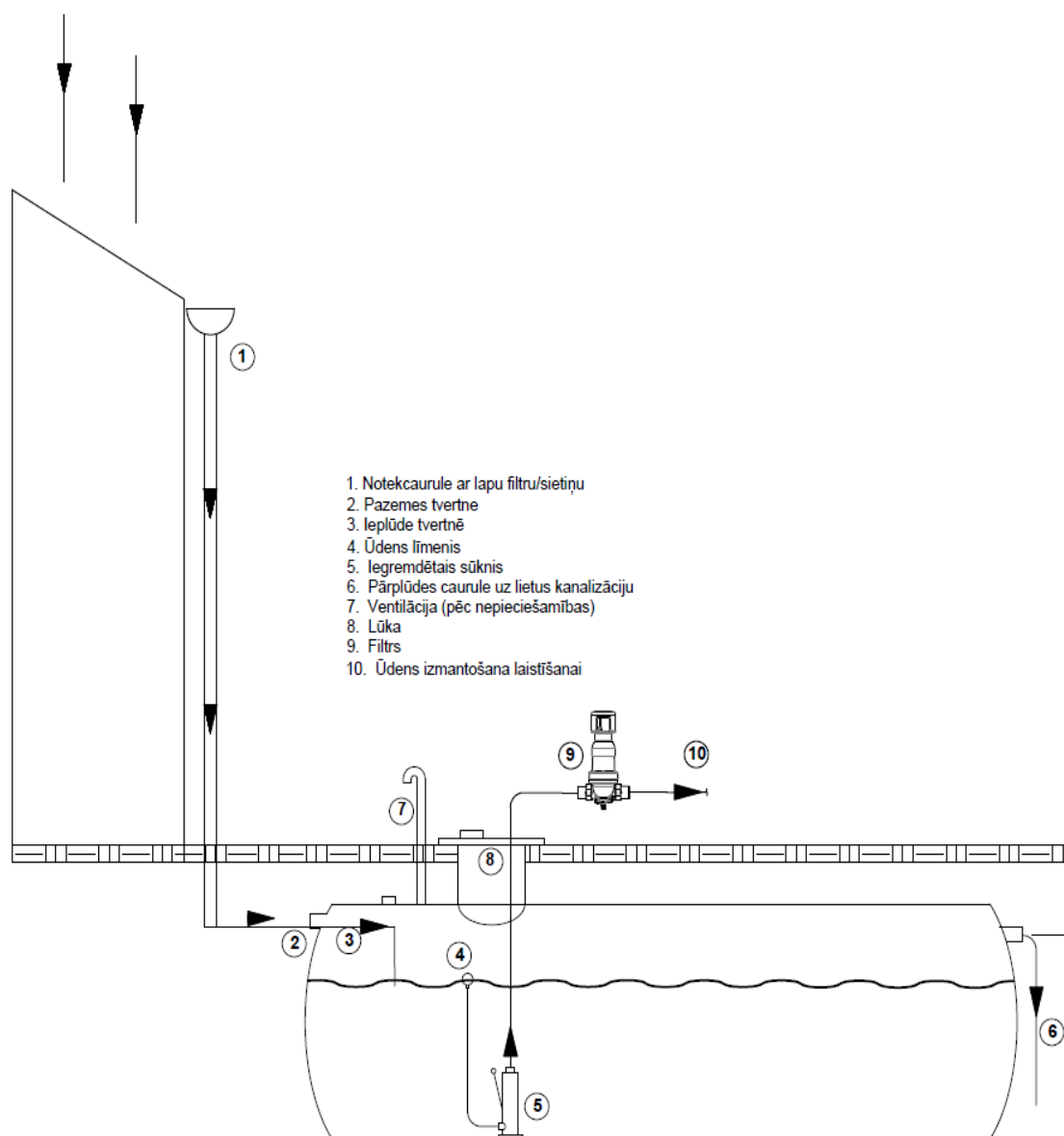
88. attēls. Shematisks piemērs risinājumam lietus ūdens izmantošanai laistīšanas vajadzībām ar pazemes rezervuāru.
