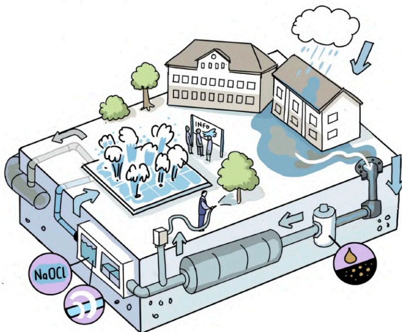
40. attēls. Lietus ūdens izmantošana Saldus novadā (avots: Euroregion Baltic Water Recycling Toolbox).
