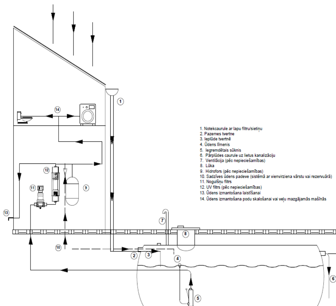
87. attēls. Shematiskis piemērs risinājumam lietus ūdens izmantošanai no pazemes tvertnes.
