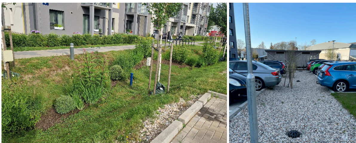
45. attēls. Bioievalka un infiltrācijas tranšeja Turaidas ielas kvartālā (foto: Jurijs Kondratenko, Krišs Maļinovskis).
